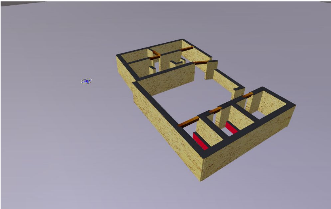
Los Almadenes. Edificio 1. Recreación volumétrica.
